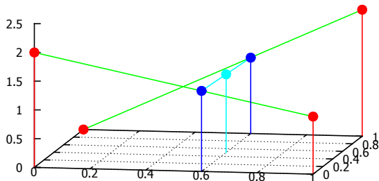
Figure: z(0.6, 0.5) érték meghatározása egydimenziós interpolálások segítségével.
