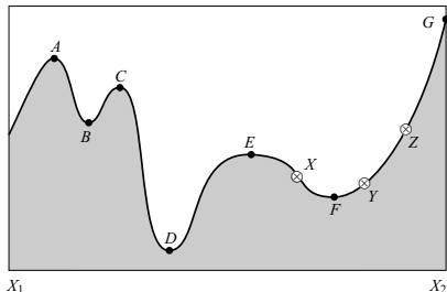
Figure: Egy függvény lokális és globális minimumai. ©Numerical Recipes
